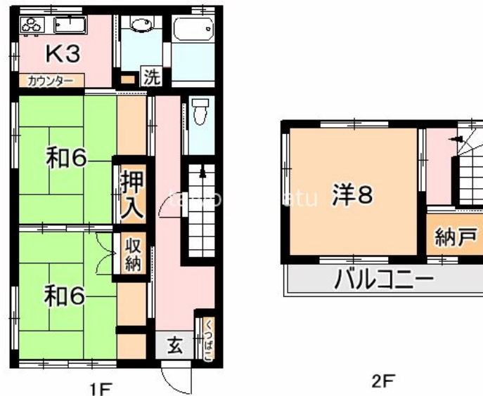
【間取り図】
